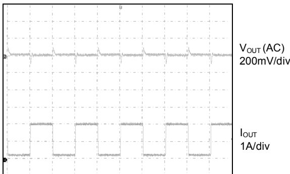
Time Base: 1ms/div
