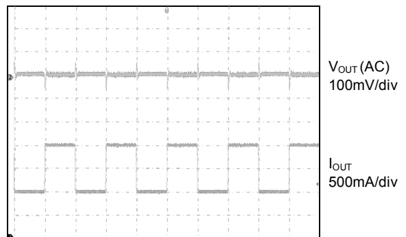
Time Base: 1ms/div
